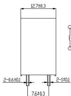
BOTTOM VIEW (1A)
