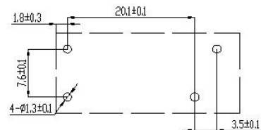
BOTTOM VIEW (1A)
